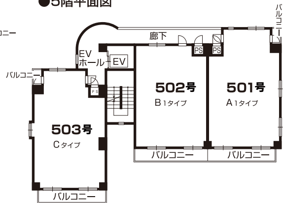
●5階平面図
