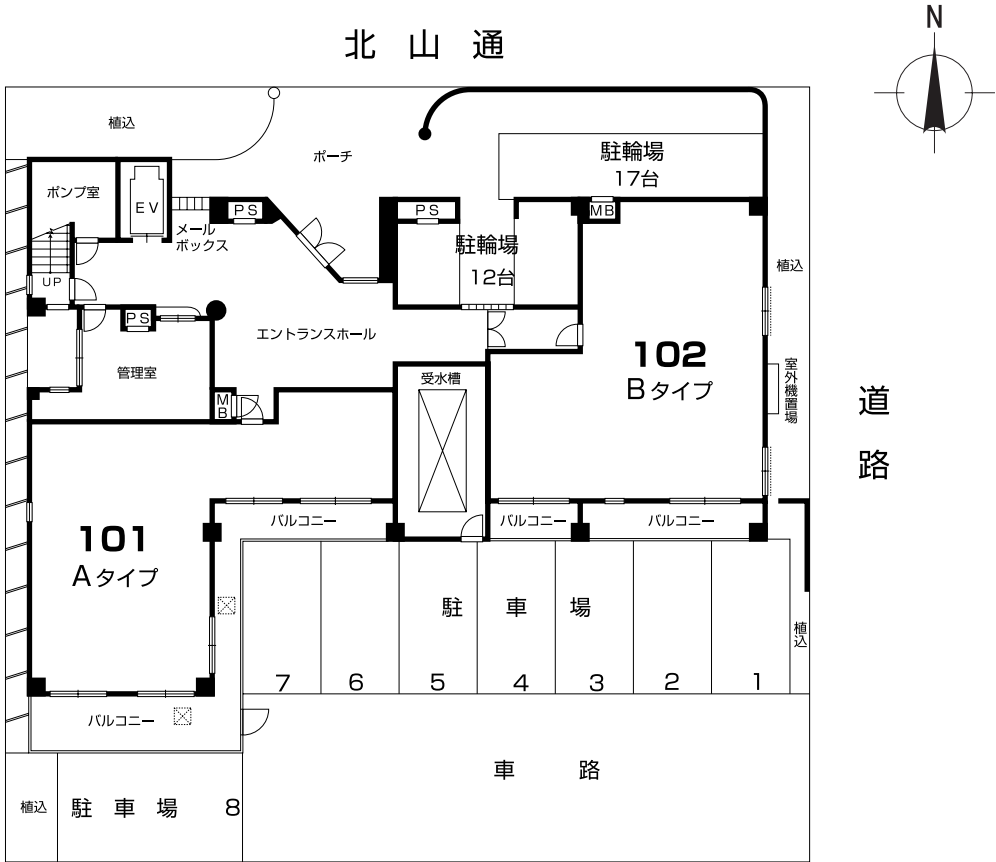
●1階平面図
