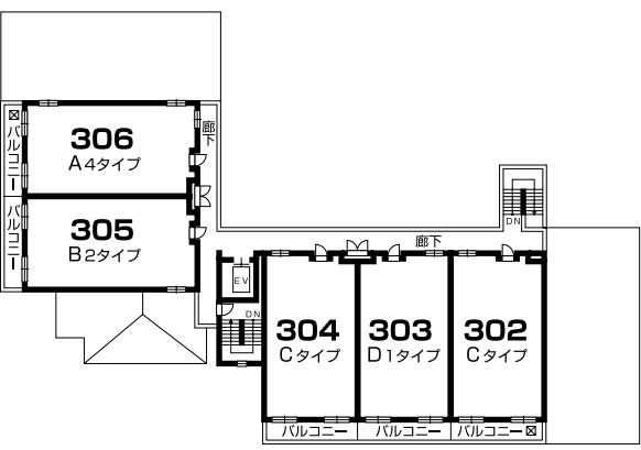
●3階平面図
