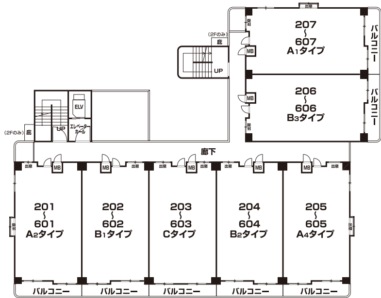
●2～6階平面図
