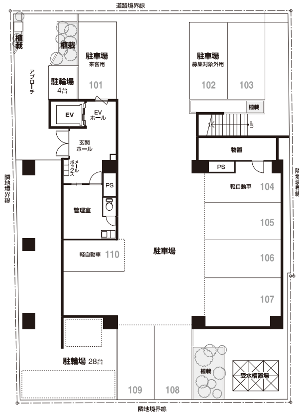
●1階平面図
