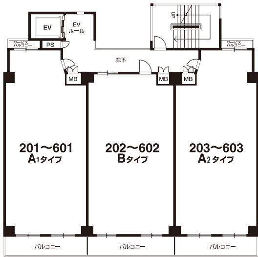
●2～6階平面図
