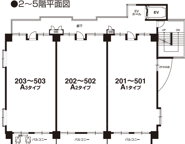
●2～5階平面図
