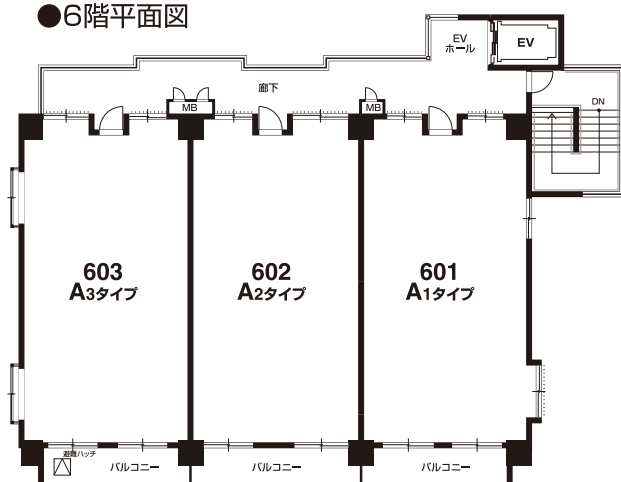
●6階平面図
