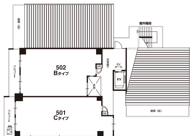
●5階平面図
