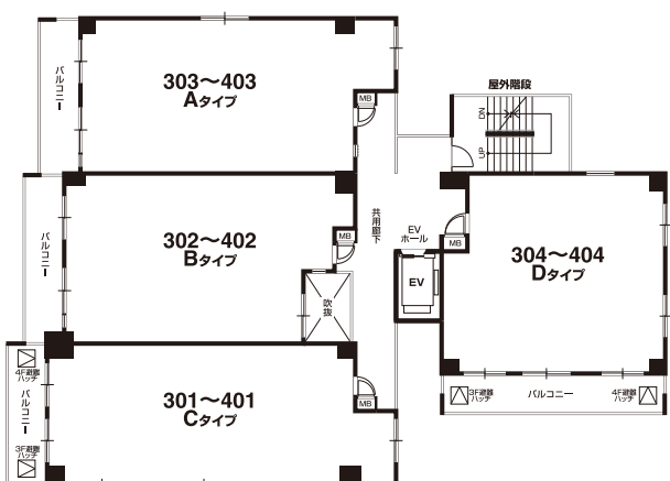
●3～4階平面図
