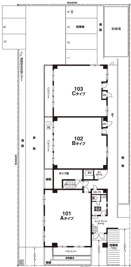
●1階平面図
