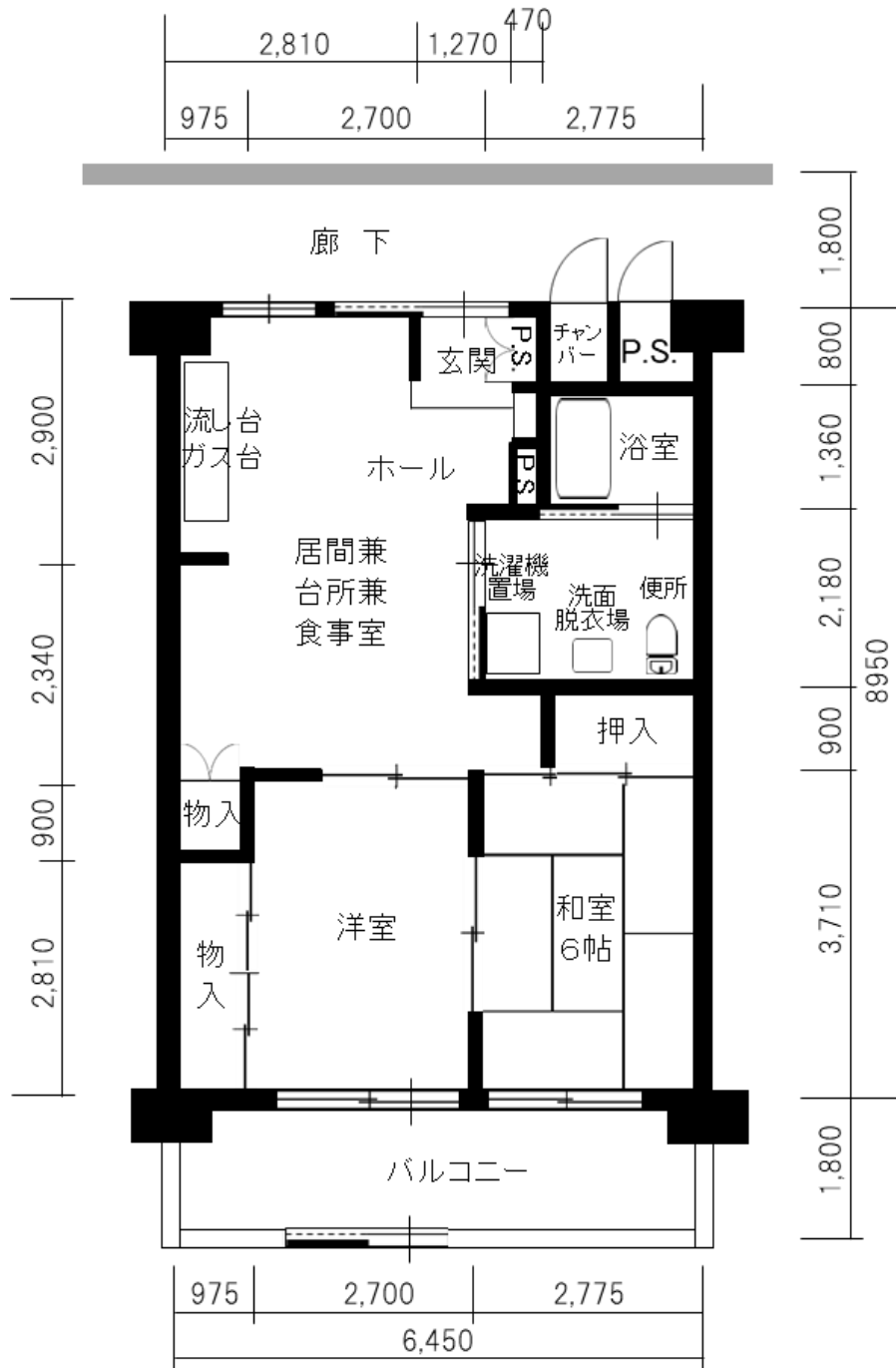
【 向島8街区 車いす住宅 標準間取り図 】
