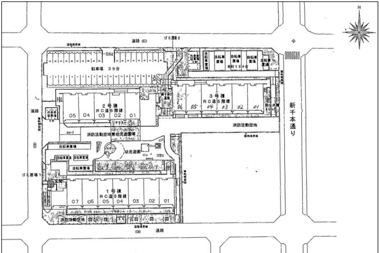
【 唐橋団地配置図 】
