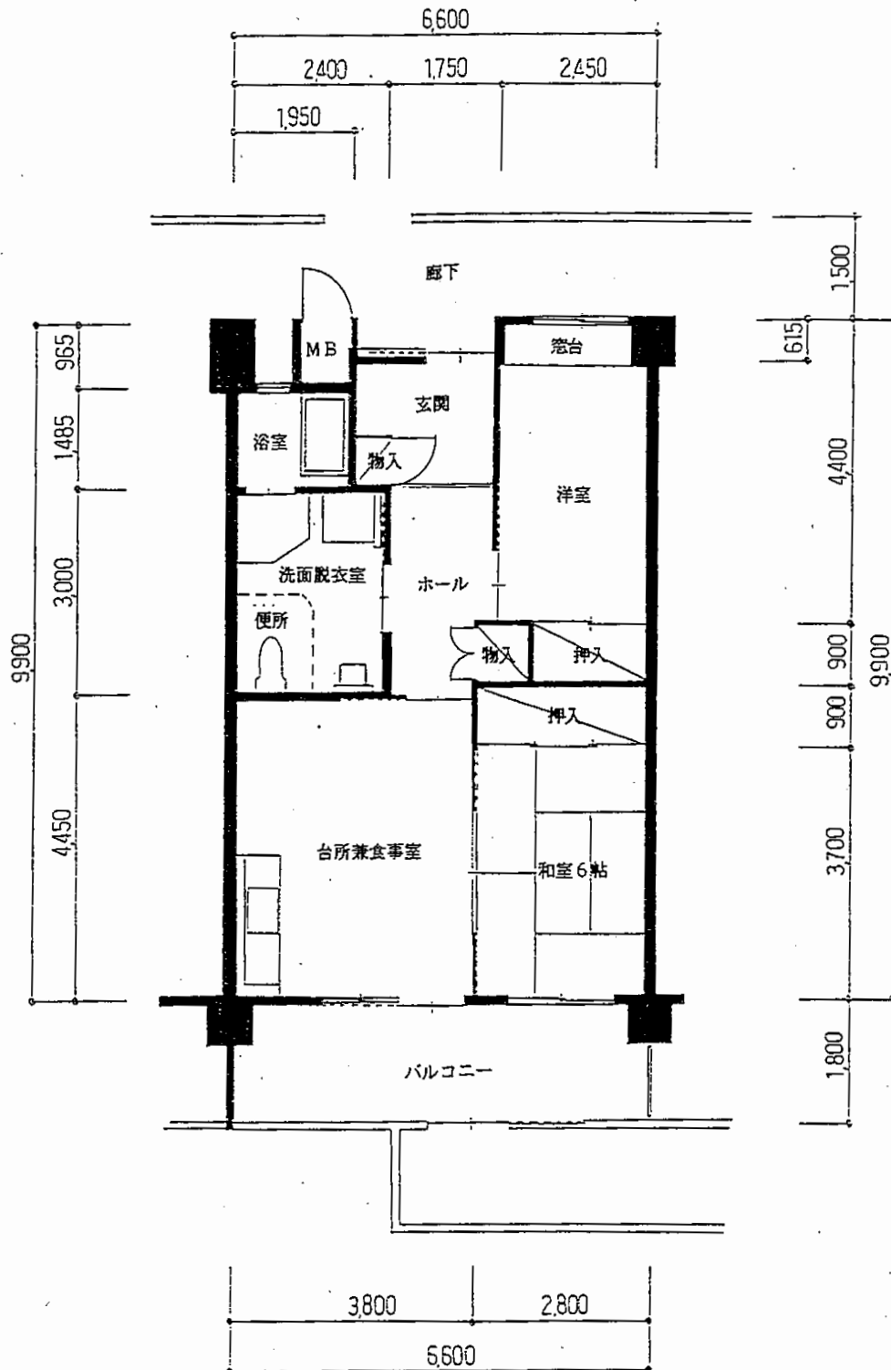
【 勸修寺第一 車いす住宅 標準間取り図 】
