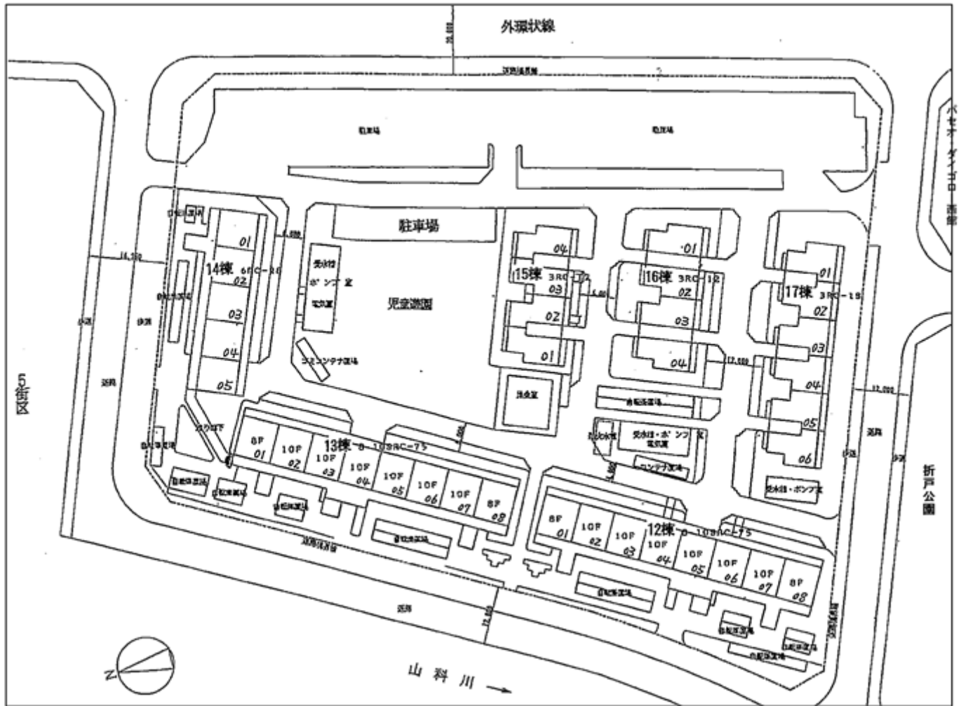
【 醍醐西 4 街区団地配置図 】
