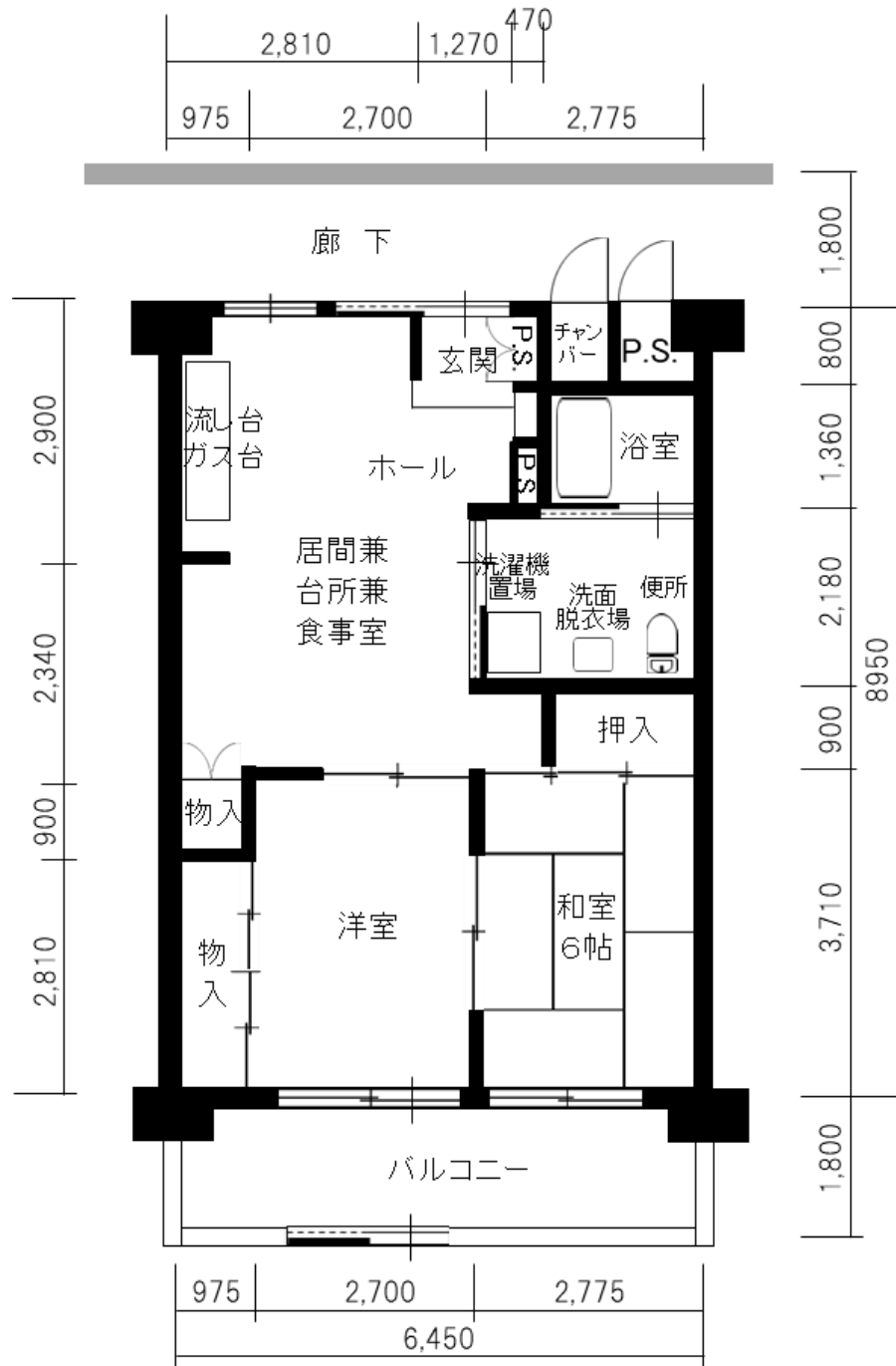
【 向島 1 0 街区 車いす住宅 標準間取り図 】
